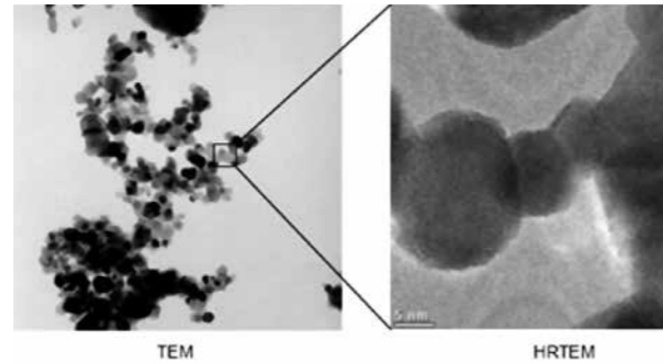
Particolare delle particelle del fotocatalizzatore (microscopio elettronico a trasmissione)
